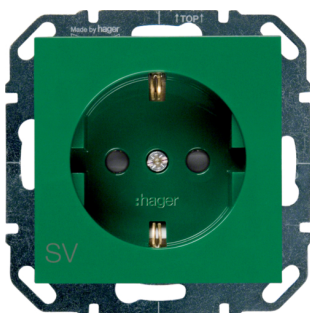
WYS404
